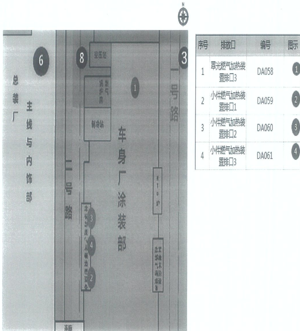
福戴二工厂加热装置废气排放口平面图 - 一般排放口 (4个, 共63个)
